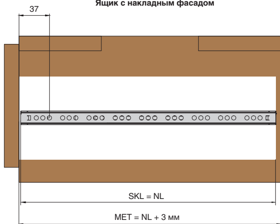
Ящик с накладным фасадом
