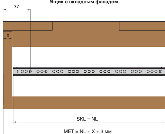
Ящик с вкладным фасадом
