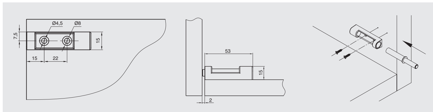
Push-Latch 14 защелка накладная с амортизатором
