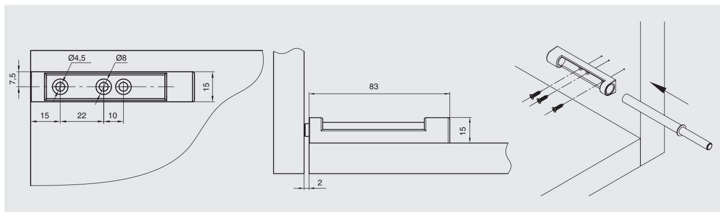
Push-Latch 37 защелка накладная с амортизатором
