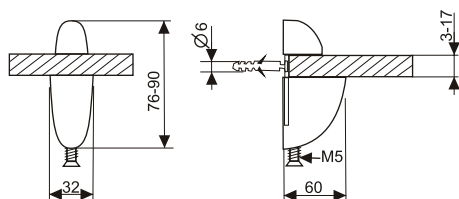
менсолдержатель пеликан прозрачный малый (комплект 2 шт.)
