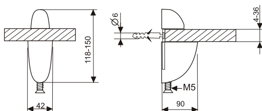
менсолдержатель пеликан прозрачный большой (комплект 2 шт.)
