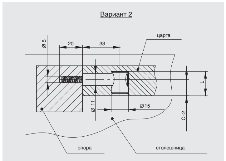
ПРИМЕР СБОРКИ СТОЛА С ПОМОЩЬЮ КОНИЧЕСКОЙ СТЯЖКИ XS
