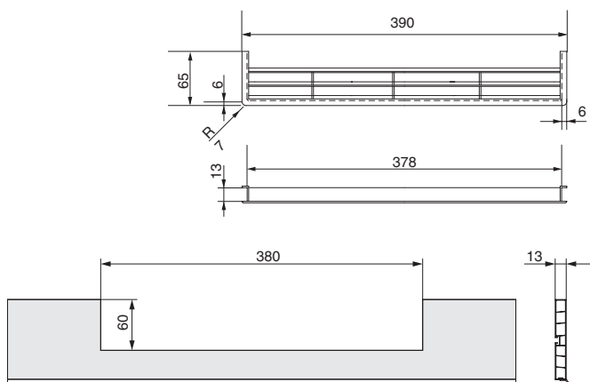
21\90.449.AV вентиляционная решётка для цоколя ПВХ
