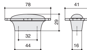
керамическая вставка
