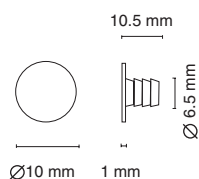
*PUSH-LATCH ответная часть d=10мм на бобышке 6.5мм
