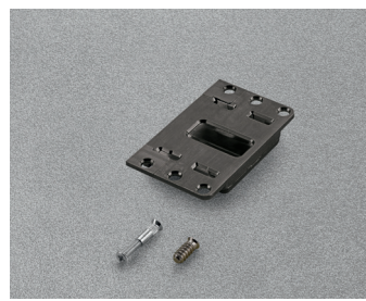
арт. DQG5BX6XI Сопеста адаптер накладной для петли скрытой (наложение 14 мм), отделка титаниум
