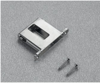
арт. DQG3BX9XI Conecta адаптер врезной для петли скрытой (наложение 16,5мм), отделка никель
