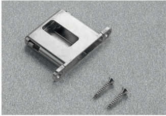
арт. DQG3BX9XI Сопеста адаптер врезной для петли скрытой (наложение 16,5мм), отделка никель
