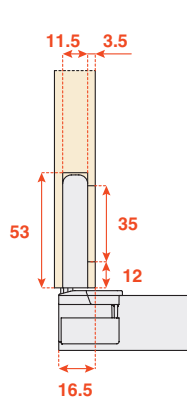
арт. CQA3KE9XXI Сопеста петля скрытая для глухих фасадов, отделка никель
