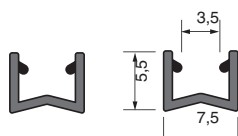
V0446C53U уплотнитель пластиковый для стекла 4мм
