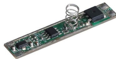
HW.012.AD003 выключатель сенсорный с диммером для алю. профилей (пружина 10 мм), 60W/12V, 120W/24V
