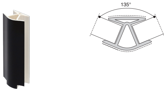
угол 135° двухсторонний
