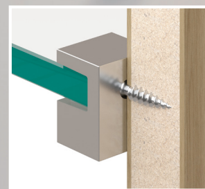
Полкодержатель под шуруп
