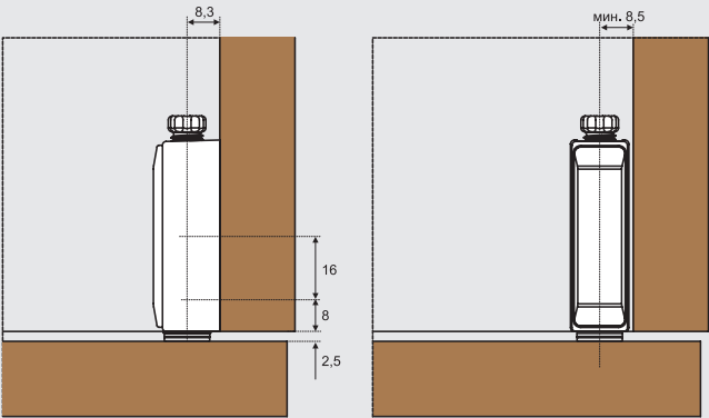
Схема накладной установки с использованием прямоугольного адаптера.
