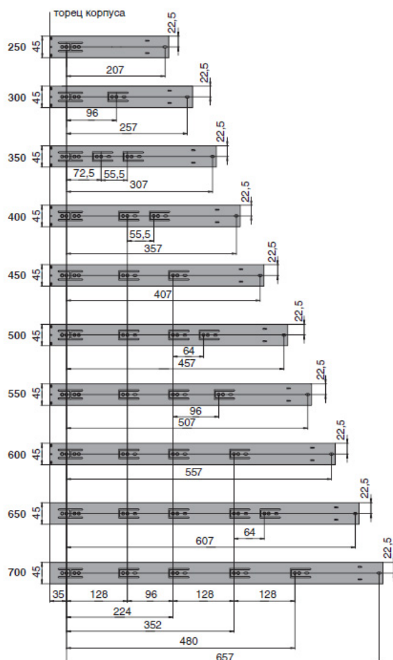
Схема крепления направляющих к корпусу
