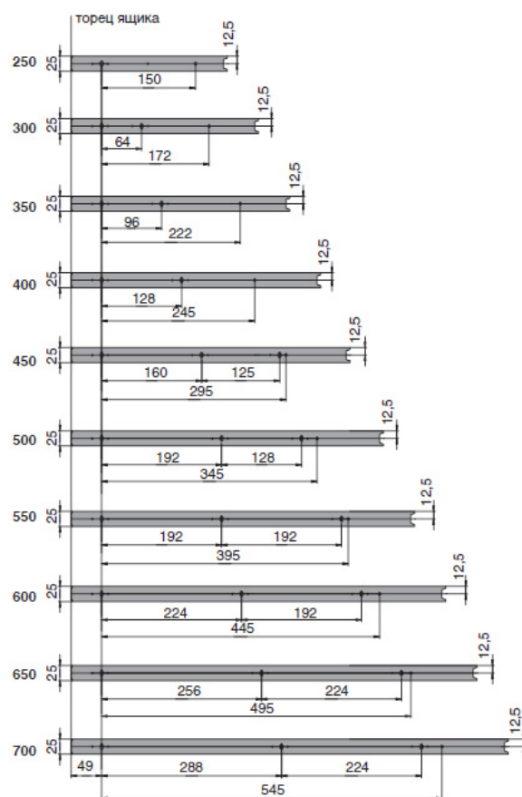
Схема крепления направляющих к каркасу ящика
