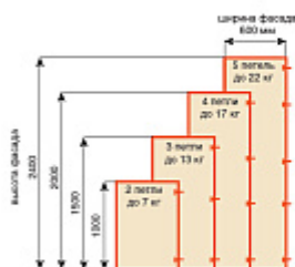
График выбора количества петель в зависимости от высоты, ширины и веса фасада
