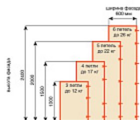
График выбора количества петель в зависимости от высоты, ширины и веса фасада
