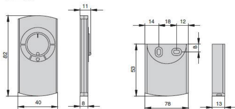
Пульт ДУ
