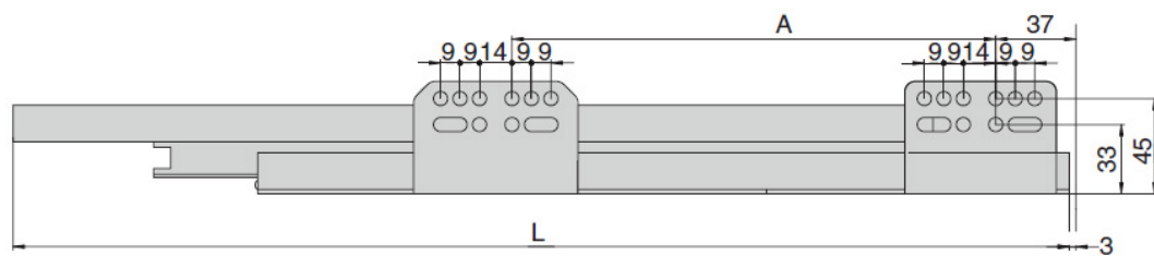
Торец каркаса
