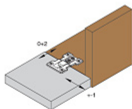
Регулировка по ширине караса и глубине
