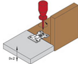
Регулировка по вертикали (высота)
