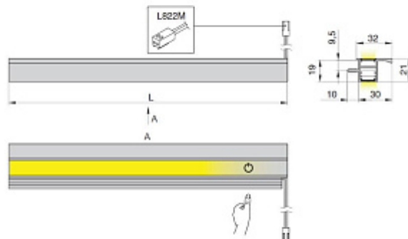
ГАБАРИТНЫЕ И УСТАНОВОЧНЫЕ РАЗМЕРЫ
