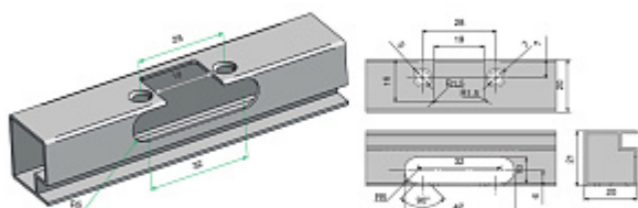
Схема привода замка накладной петли для узкого алюминиевого профиля шириной 20-21 мм
