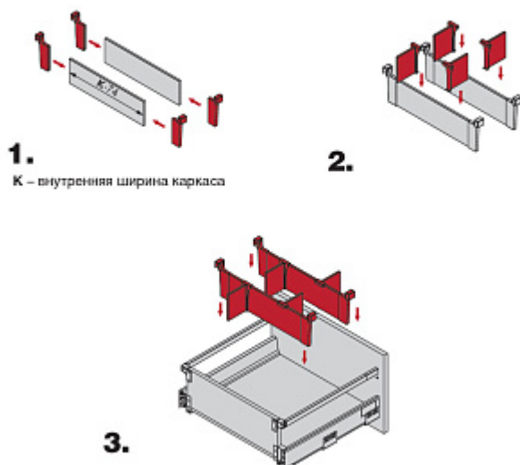
Установка профиль-делителя
