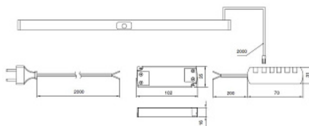
СХЕМА ПОДКЛЮЧЕНИЯ ДЛЯ KIT1
