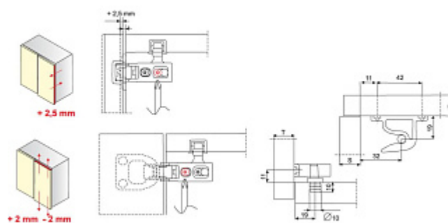
Схема регулировки
