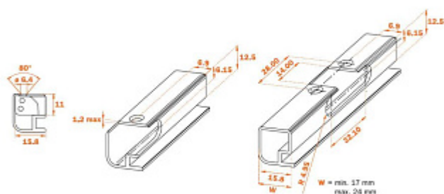
Схема присадки пелли с обратной пружиной для узкого алюминиевого профиля шириной 17-24 мм
