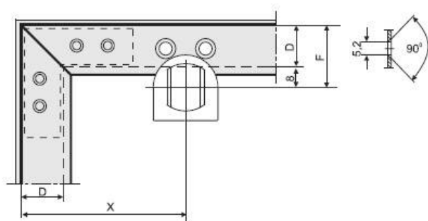
схема присадки системы PUSH для алюминиевых рамок 17-35 мм шириной
