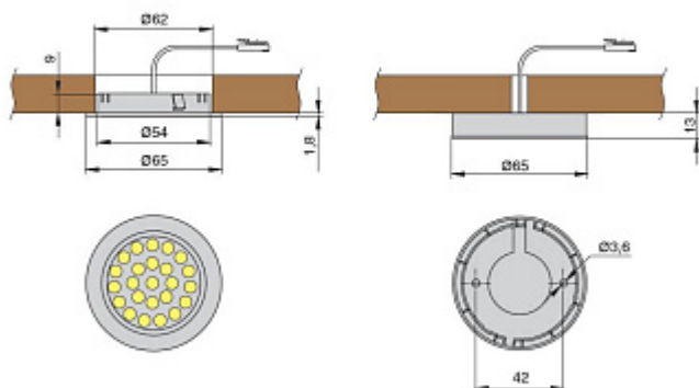
ГАБАРИТНЫЕ И УСТАНОВОЧНЫЕ РАЗМЕРЫ
