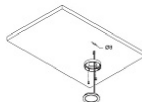
Вариант 2 Накладной с использованием расширителя
