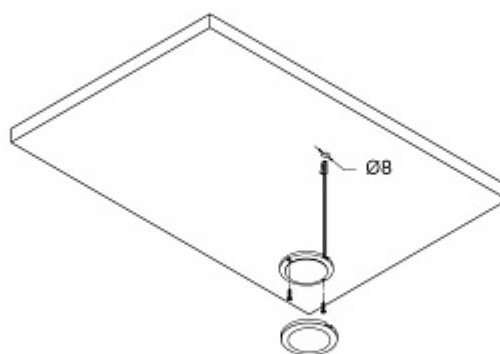
Схема монтажа:
