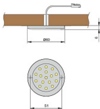
ГАБАРИТНЫЕ И УСТАНОВОЧНЫЕ РАЗМЕРЫ
