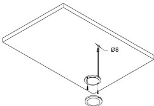
Схема монтажа:
