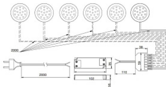
СХЕМА ПОДКЛЮЧЕНИЯ ДЛЯ КИТ1, КИТ2, КИТ3, КИТ4, КИТ5, КИТ6
