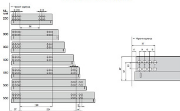
Позиция креплений направляющих к корпусу
