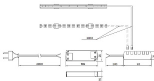
СХЕМА ПОДКЛЮЧЕНИЯ ДЛЯ КИТ1, КИТ2
