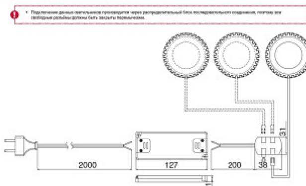
СХЕМА ПОДКЛЮЧЕНИЯ ДЛЯ KIT1, KIT2, KIT3
