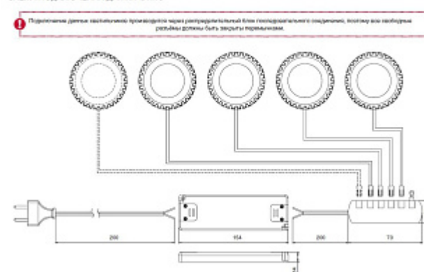
СХЕМА ПОДКЛЮЧЕНИЯ ДЛЯ KIT4, KIT5
