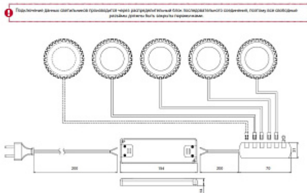
СХЕМА ПОДКЛЮЧЕНИЯ ДЛЯ KIT4, KIT5
