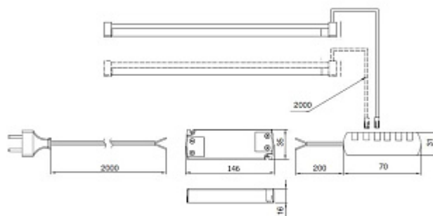
СХЕМА ПОДКЛЮЧЕНИЯ ДЛЯ KIT1, KIT2
