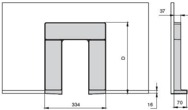
Габаритные размеры
