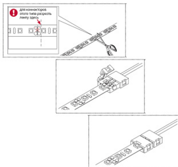
СХЕМА МОНТАЖА И ПОДКЛЮЧЕНИЯ КОННЕКТОРА ТИП L8-1
