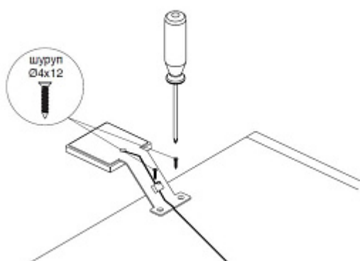
СХЕМА МОНТАЖА
