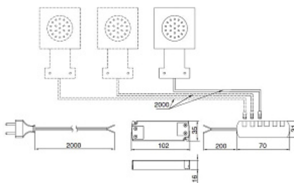
СХЕМА ПОДКЛЮЧЕНИЯ ДЛЯ КИТ1, КИТ2, КИТ3
