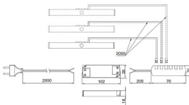
СХЕМА ПОДКЛЮЧЕНИЯ ДЛЯ KIT1, KIT2, KIT3
