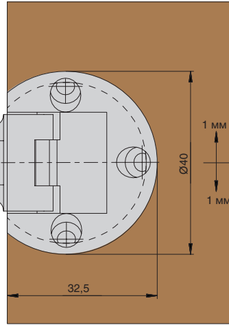
регулировка высоты
