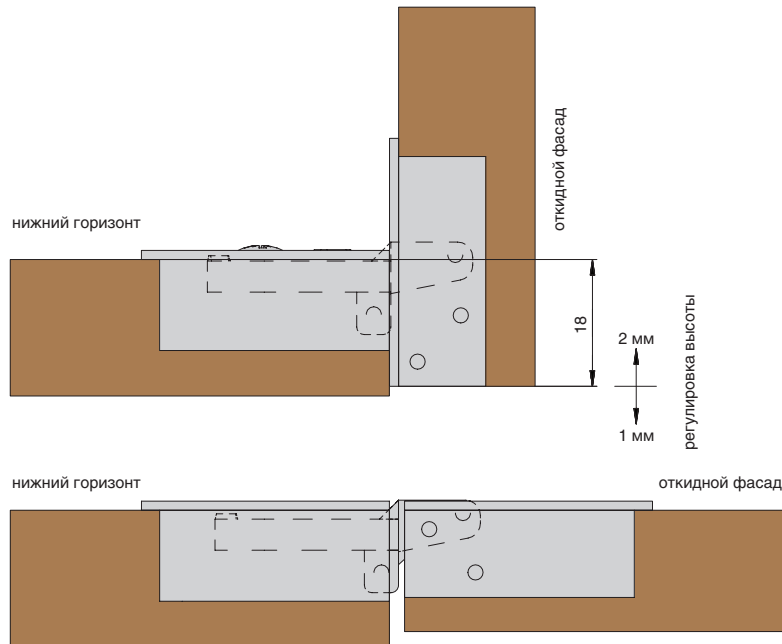
регулировка высоты
