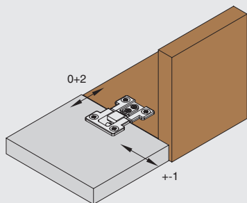
Регулировка по ширине каркаса и глубине
