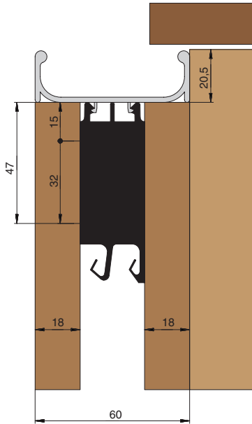
Боковая установка профиля
