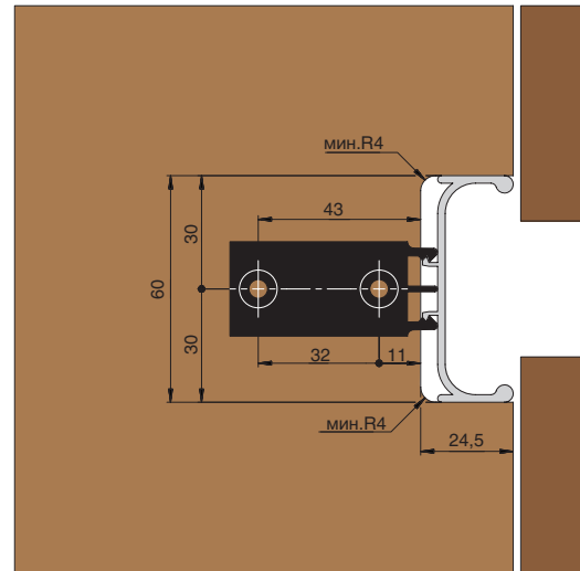
Средняя установка профиля
