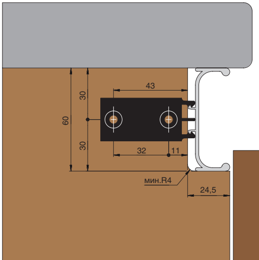
Установка профиля под столешницу
