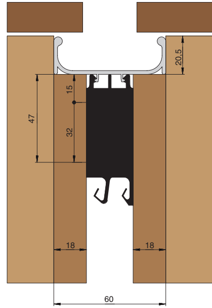
Промежуточная установка профиля
