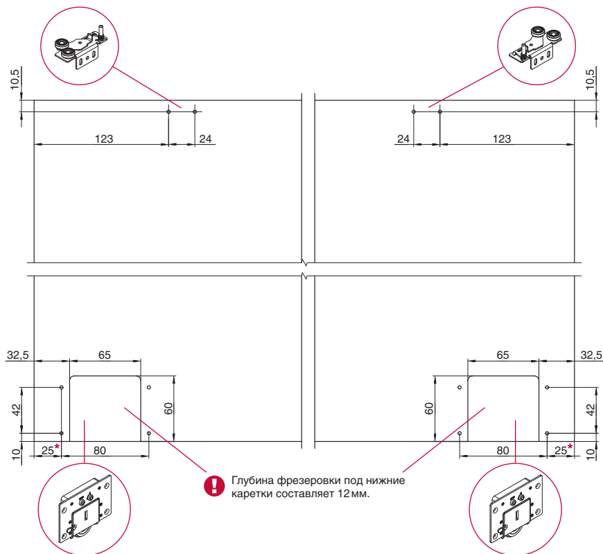
Схема присадки фасада
