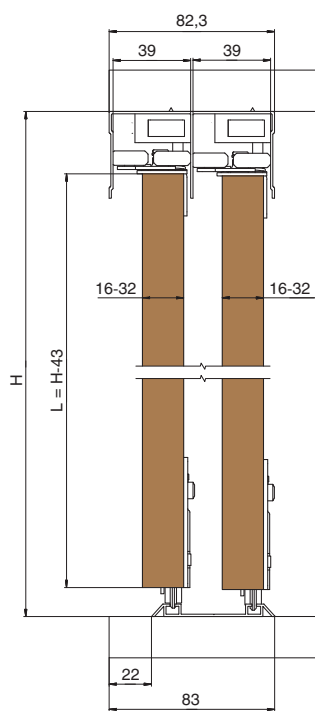
Расчет высоты фасада
