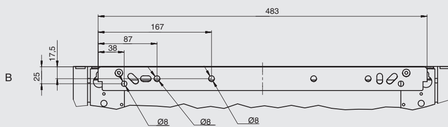
Монтажная пластина для крепления к стене
